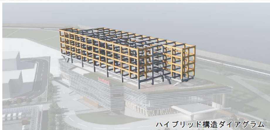
上層4フロアの外周部を木造とした魅せるハイブリッド構造
